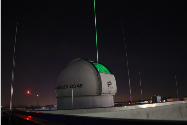
Fig. 1: Rayleigh lidar at Oberpaffenhofen.
